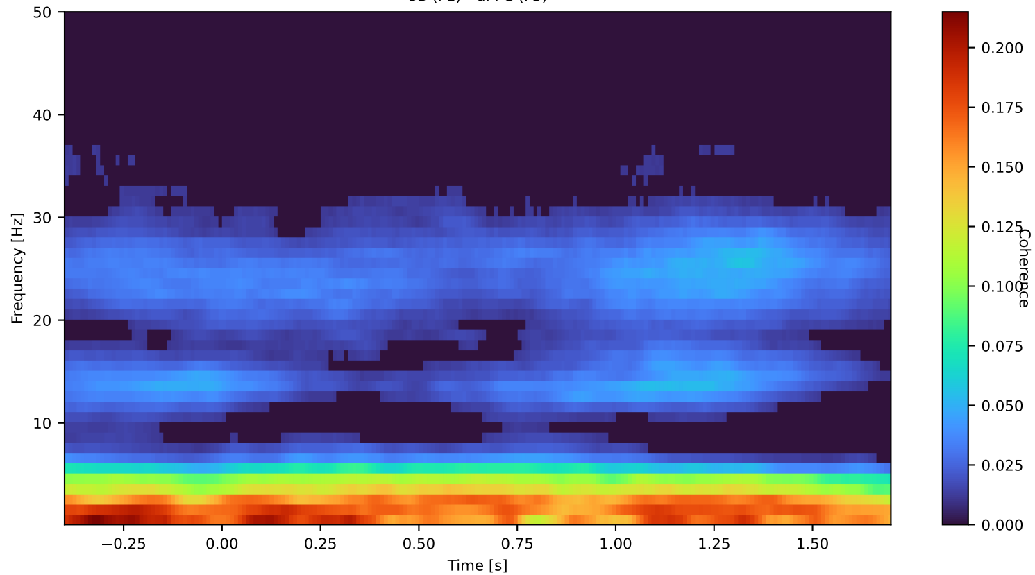
8B (F1) - dPFC (F5)
